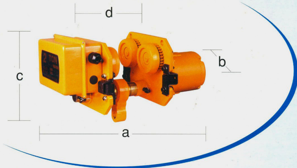
◎ 單軌電動小車規格尺寸 / USM DIMENSIONS
